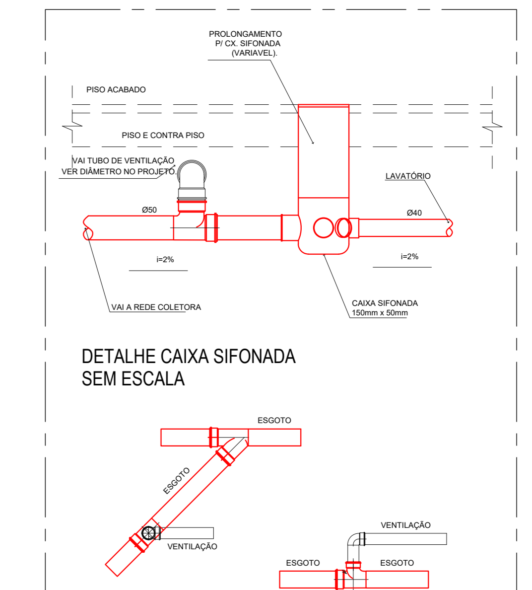
DETALHE TUBO DE VENTILAÇÃO SEM ESCALA
