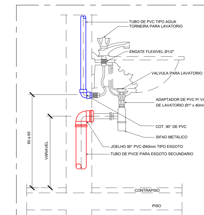
DETALHE LAVATÓRIO SEM ESCALA
