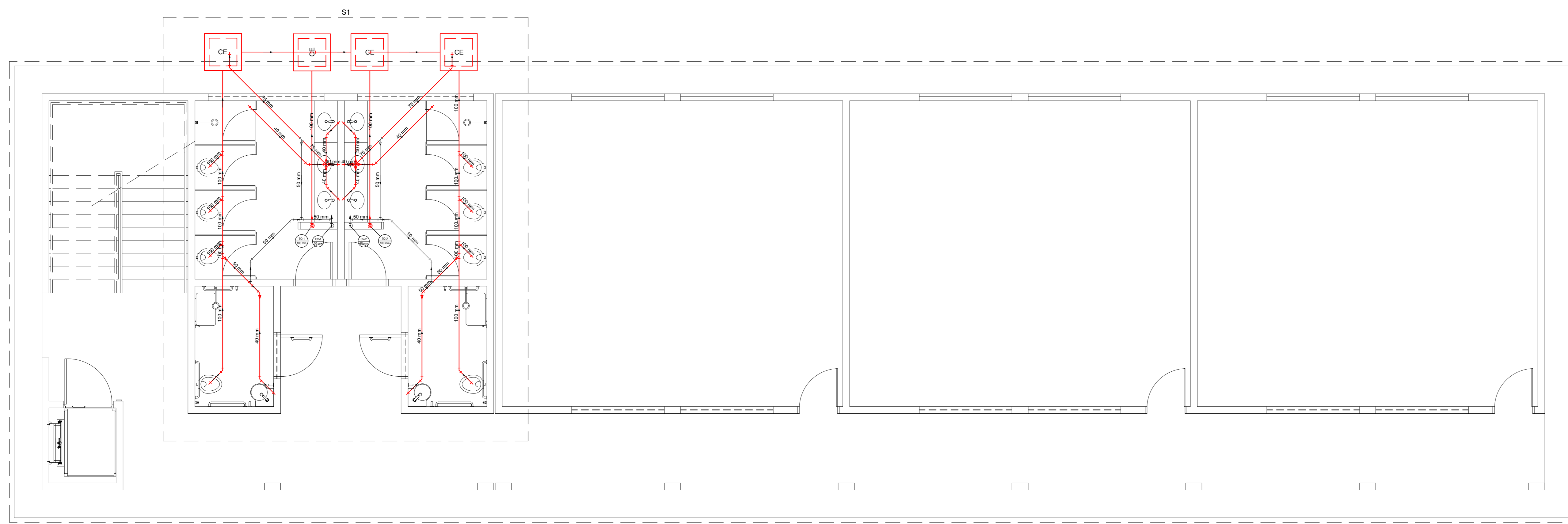
Planta do Térreo - Esgoto Escala 1:50
