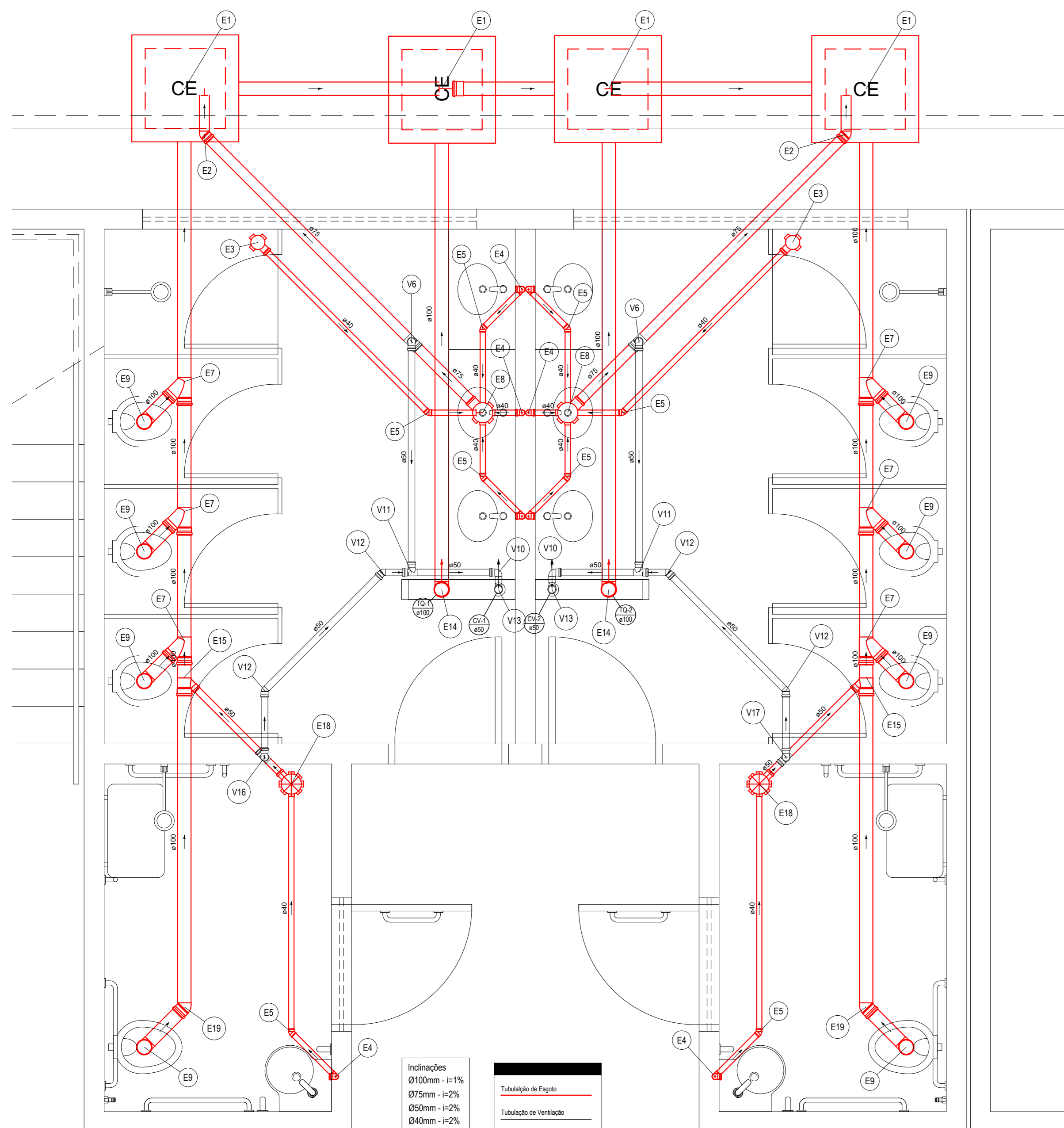
Detalhe S1 Escala 1:25
