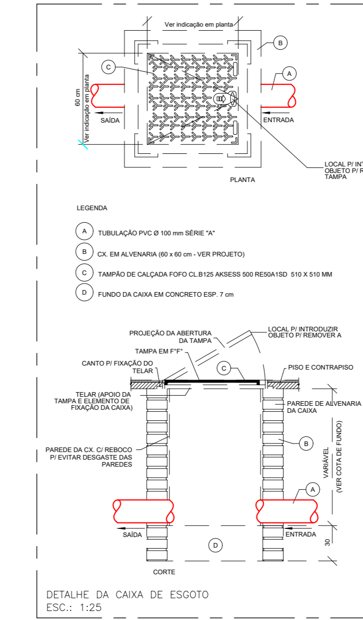
DETALHE DA CAIXA DE ESGOTO ESC.: 1:25
